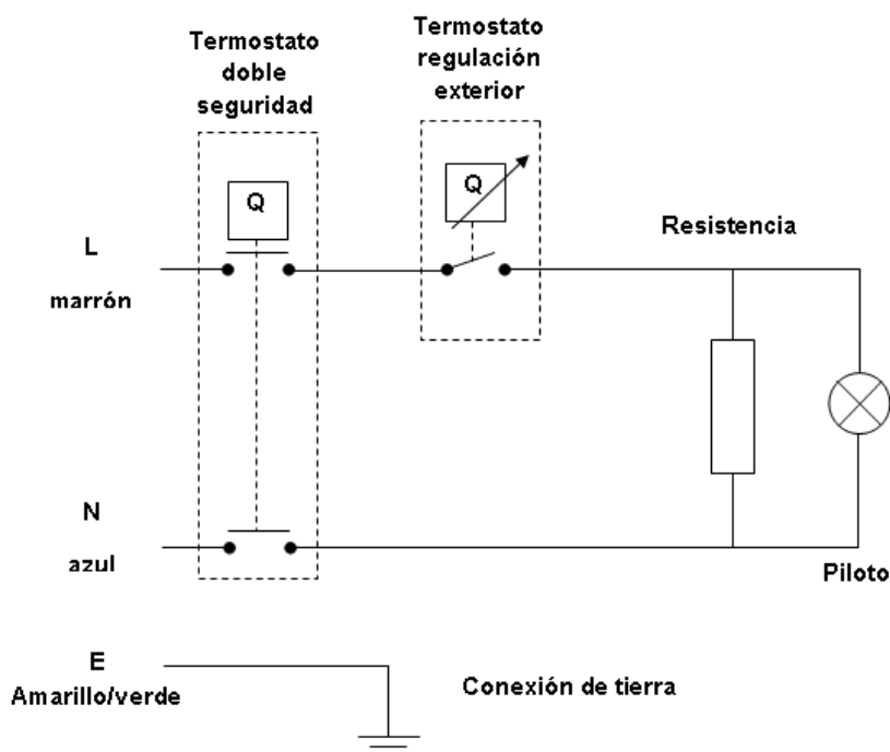
Fig. – 4 Esquema unifilar modelo NOFER – SB30C
