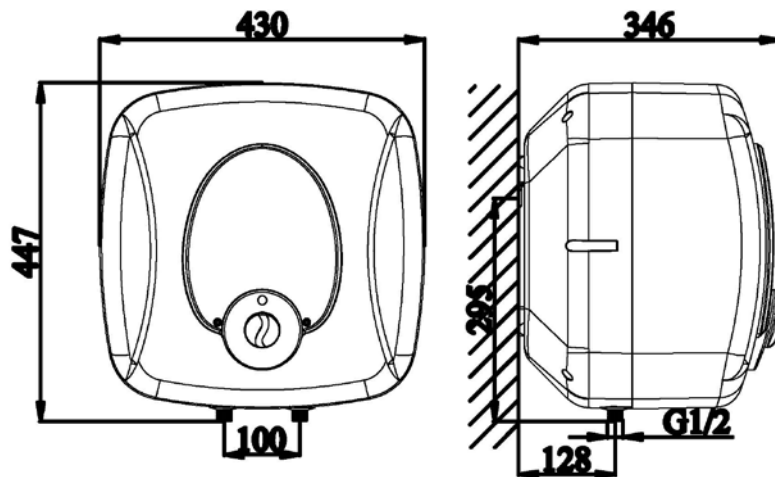
fig.-1 – Modelo NOFER SB30C
