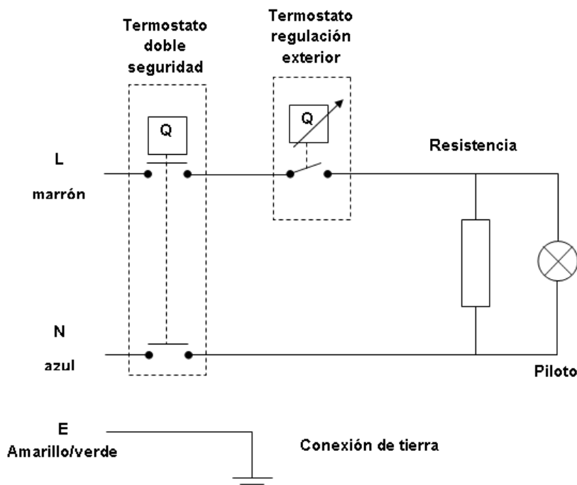
Fig. – 4 Esquema unifilar modelo NOFER – SB
