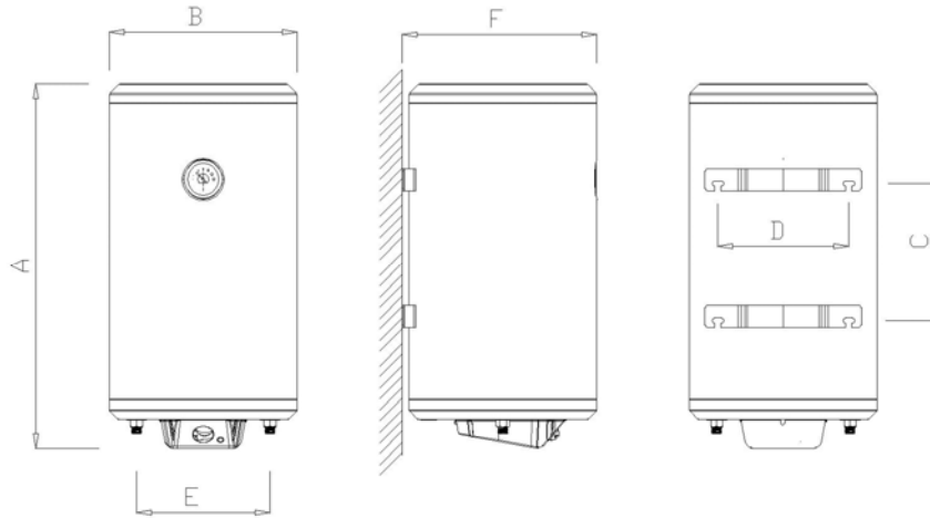
fig.-1 – Modelo NOFER SB
