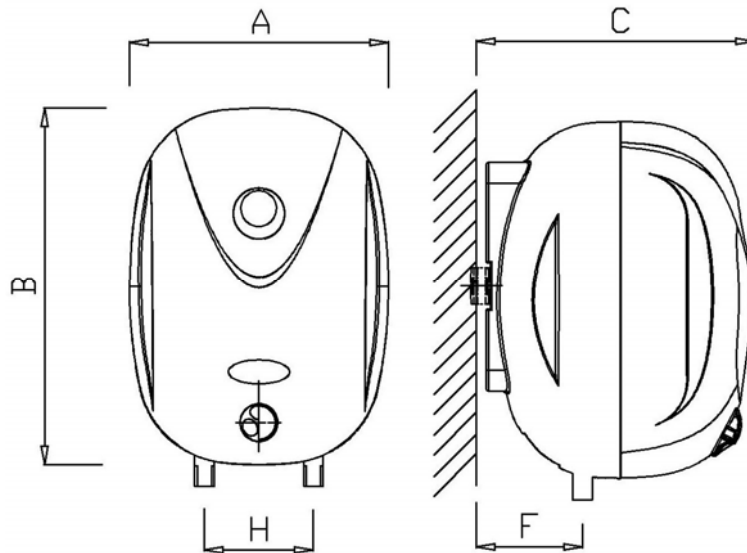
fig.-1 – Modelo NOFER SB10
