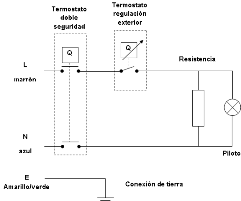
Fig. – 3 Esquema unifilar modelo NOFER – SB10
