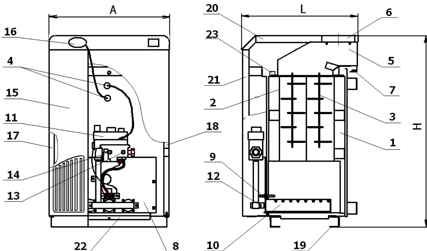
Рисунок 1. Котел отопительный стальной АОГВ-25, АКГВ-25, АОГВ-30 и АКГВ-30.
