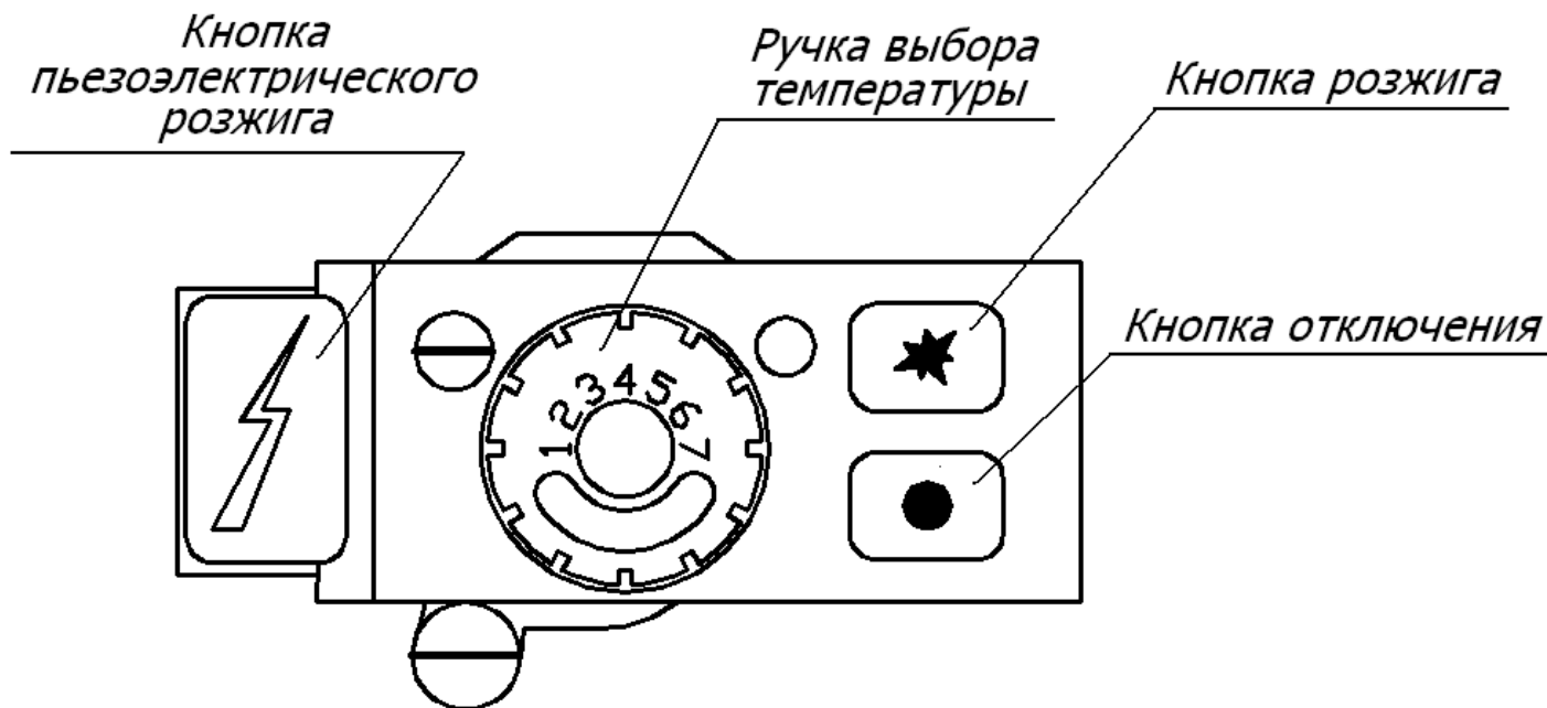
Рисунок 3. Элементы управления газового клапана 710 MINISIT.
