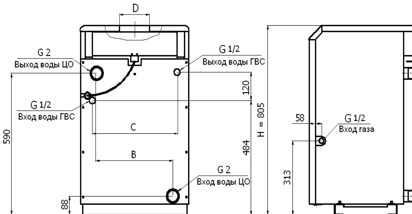
Рисунок 2. Присоединительные размеры котла отопительного стального АОГВ-25, АКГВ-25, АОГВ-30 и АКГВ-30 ( вид сзади)
